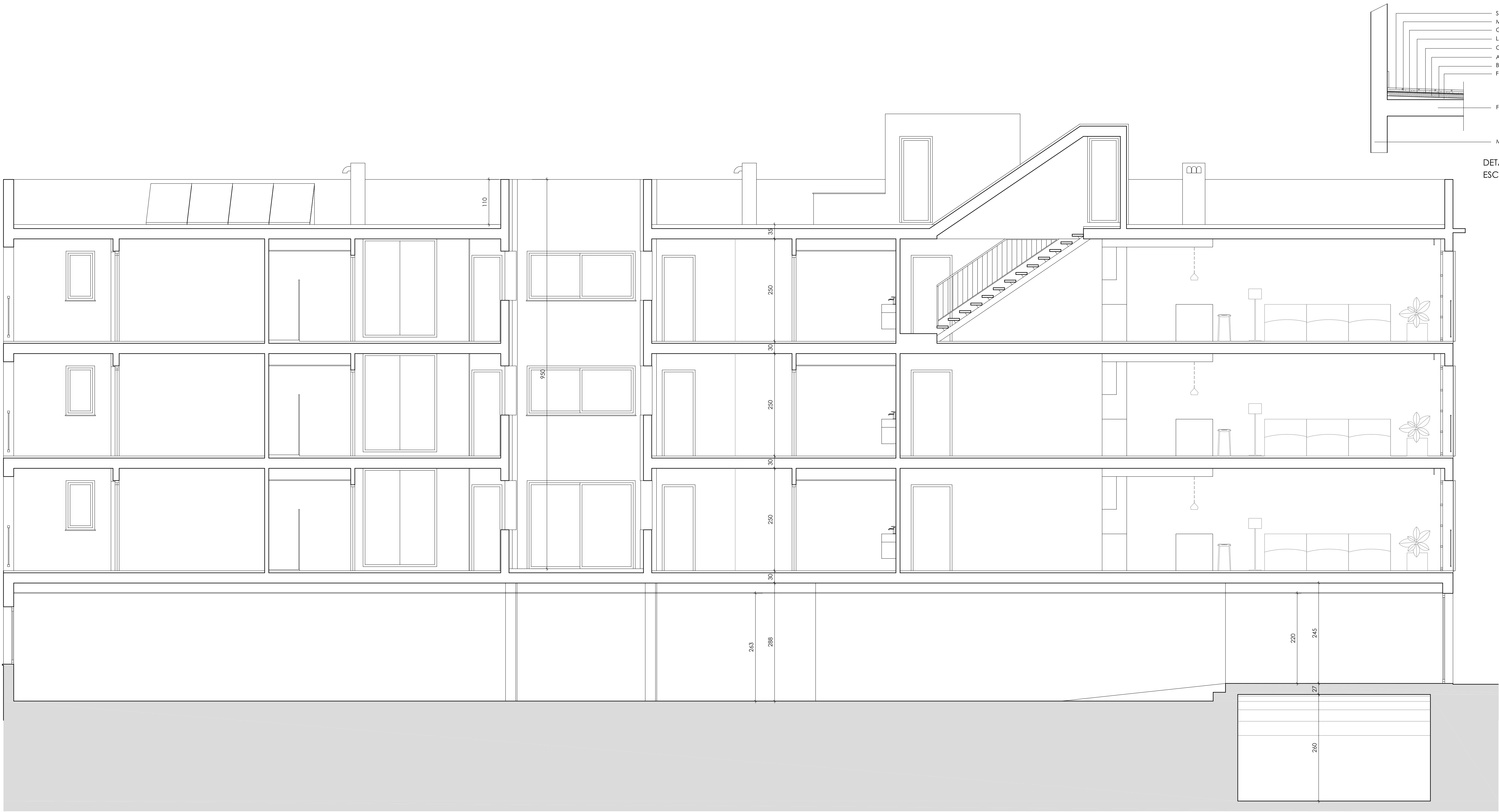
SECCION B-B'
